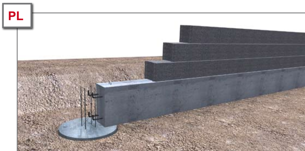
Exemple de montage de poutre lisse (PL) pour toute assise de mur (entre poteaux métalliques) ou pour longrine haute d'arrêt.
