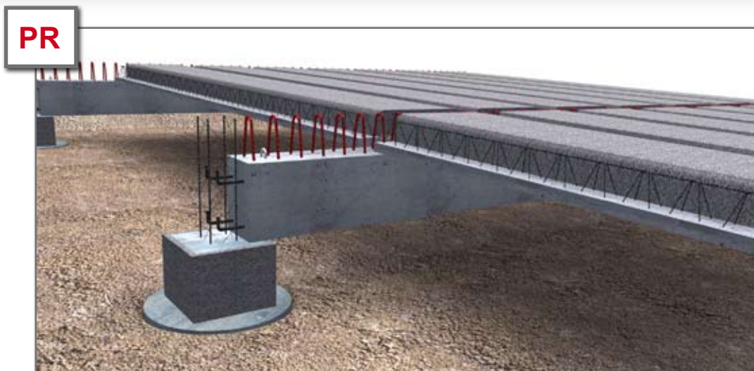
Exemple de détail d'un montage avec poutres (PR) pour VS ou de structure.
