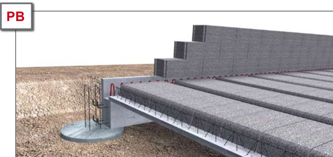
Exemple de détail d'un montage avec poutres (PB) pour rive de plancher ou butée de dallage.
